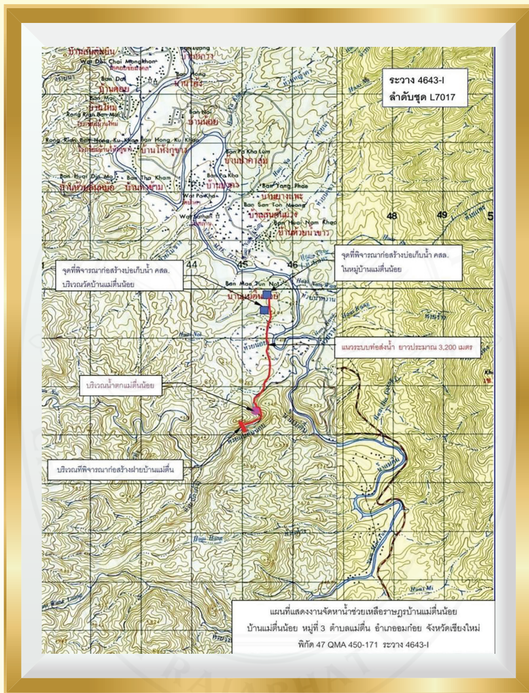
ภาพที่ ๑ แผนที่แสดงที่ตั้งโครงการ (มูลนิธิปิดทองหลังพระ, ๒๕๖๒)
